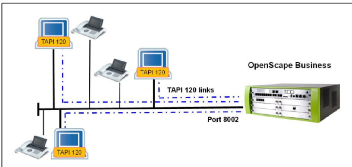
Abbildung 10: TAPI 120 im UC Smart Modus mit OpenScape Business X5R
