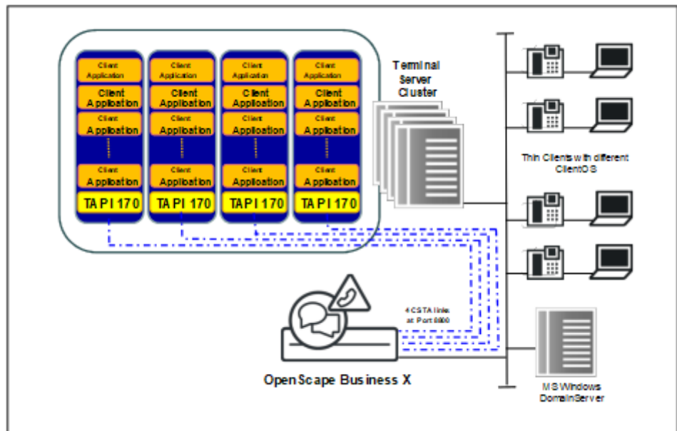
Abbildung 13: Client-basierte TAPI 170 Applikation auf Terminal-Server an OpenScape Business
