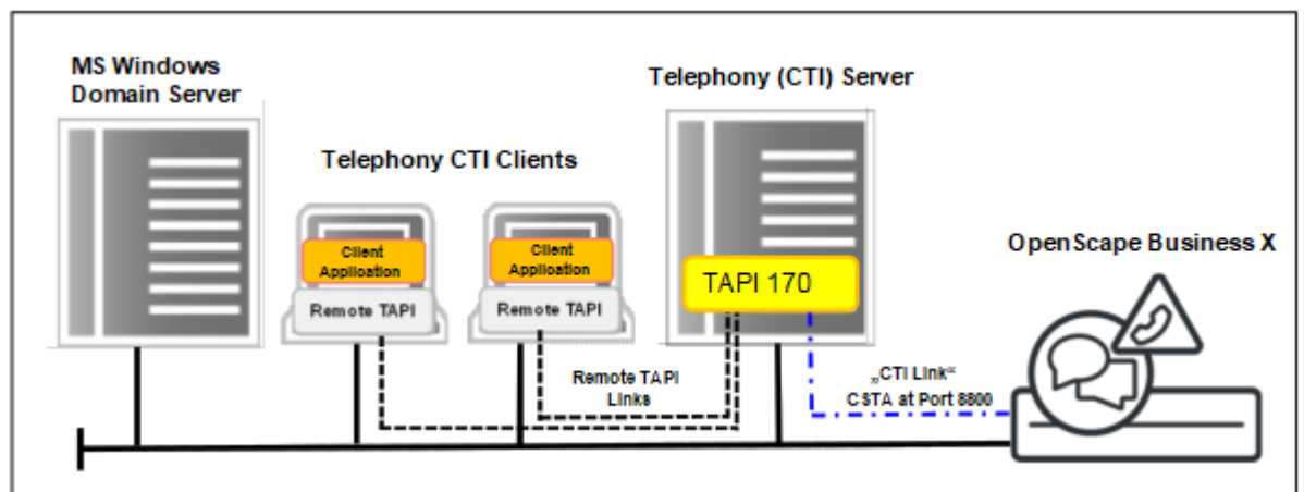
Abbildung 12: Clientbasierte TAPI-Applikation über "Remote TAPI" an OpenScape Business
