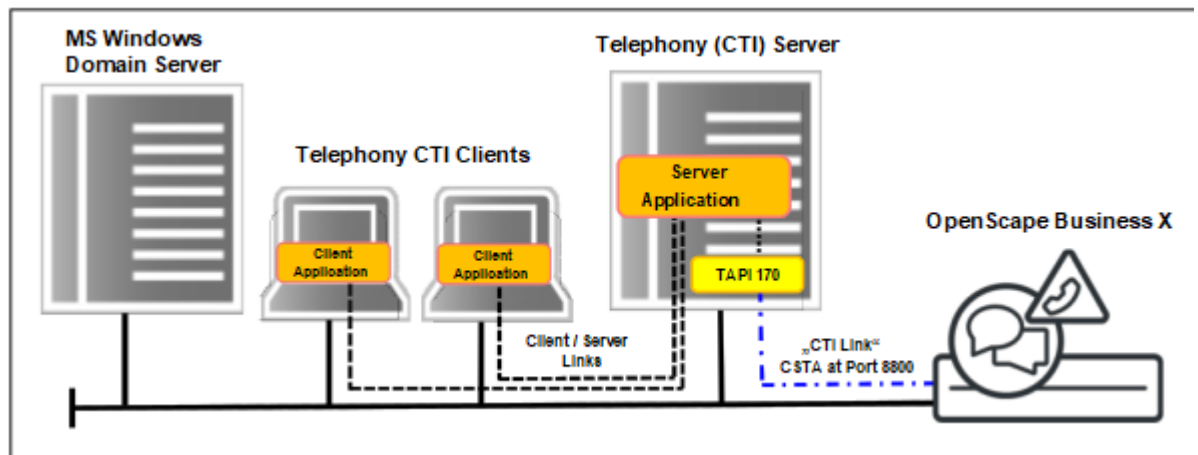
Abbildung 11: Serverbasierte TAPI-Applikation über TAPI 170 an OpenScape Business
