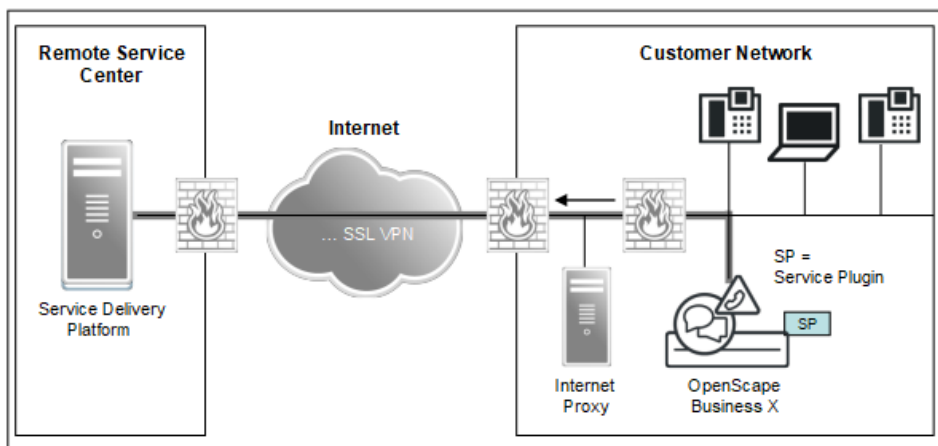
Abbildung 15: RSP - Übersicht für OpenScap Business X
