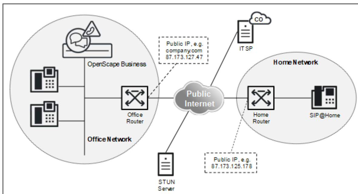
Abbildung 7: Gerät@Home (SIP-Gerät@Home- oder Systemgerät@Home-)Komponenten
