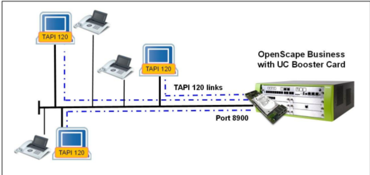
Abbildung 9: TAPI 120 im CSTA Modus mit OpenScape Business X5R und UC Booster Card
