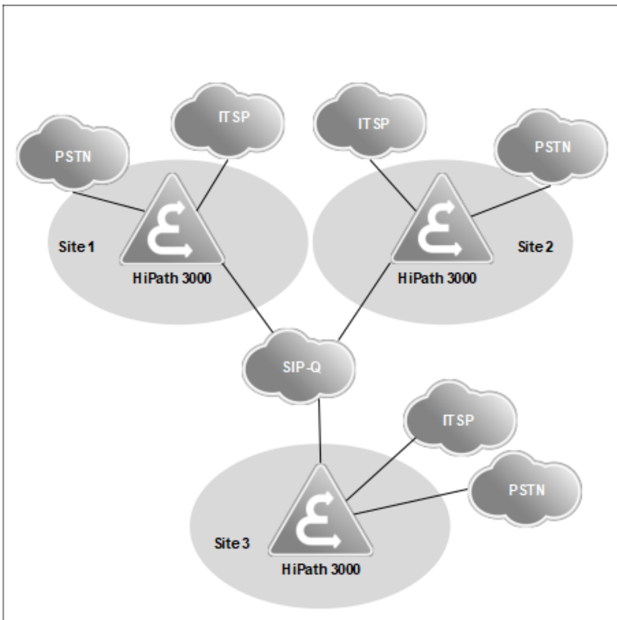
Abbildung 16: HiPath 3000 V9 Netzverbund
